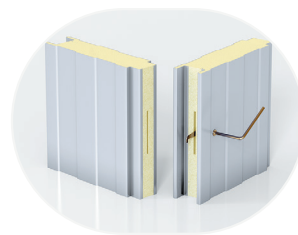
Возможна установка эксцентриковых замков
