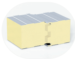
Тройной шип-паз конической формы при толщине 180 — 200 мм
