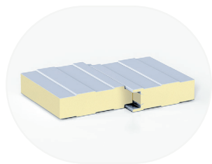
Одинарный шип-паз при толщине стеновых сэндвич-панелей 40 — 60 мм
